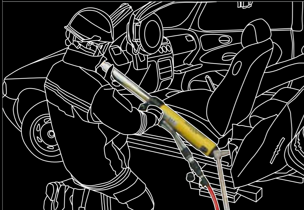
3 Rettungszyylinder ausfahren Extend rescue ram
