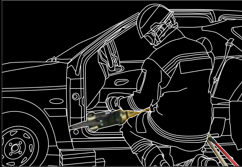
1 Entlastungsschnitte Schweller/A-Säule setzen Apply relief cut in door sill and A-pillar
